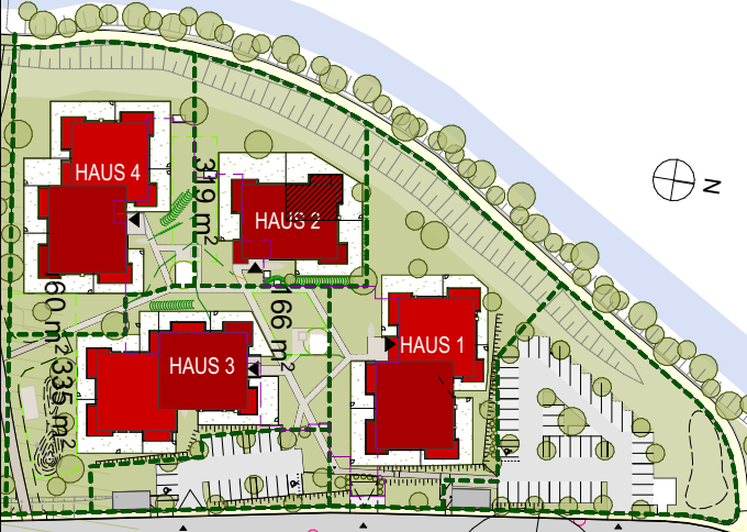
LAGEPLAN
