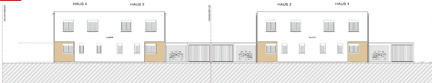
ANSICHT NORDOST
