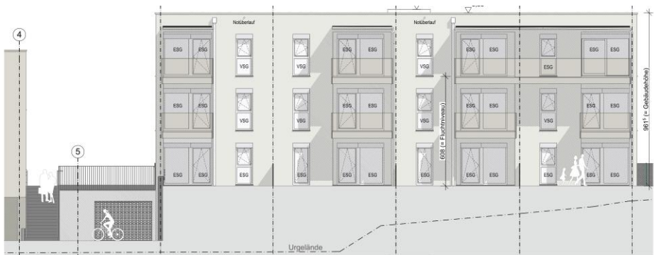
Südansicht
