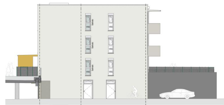
Westansicht
