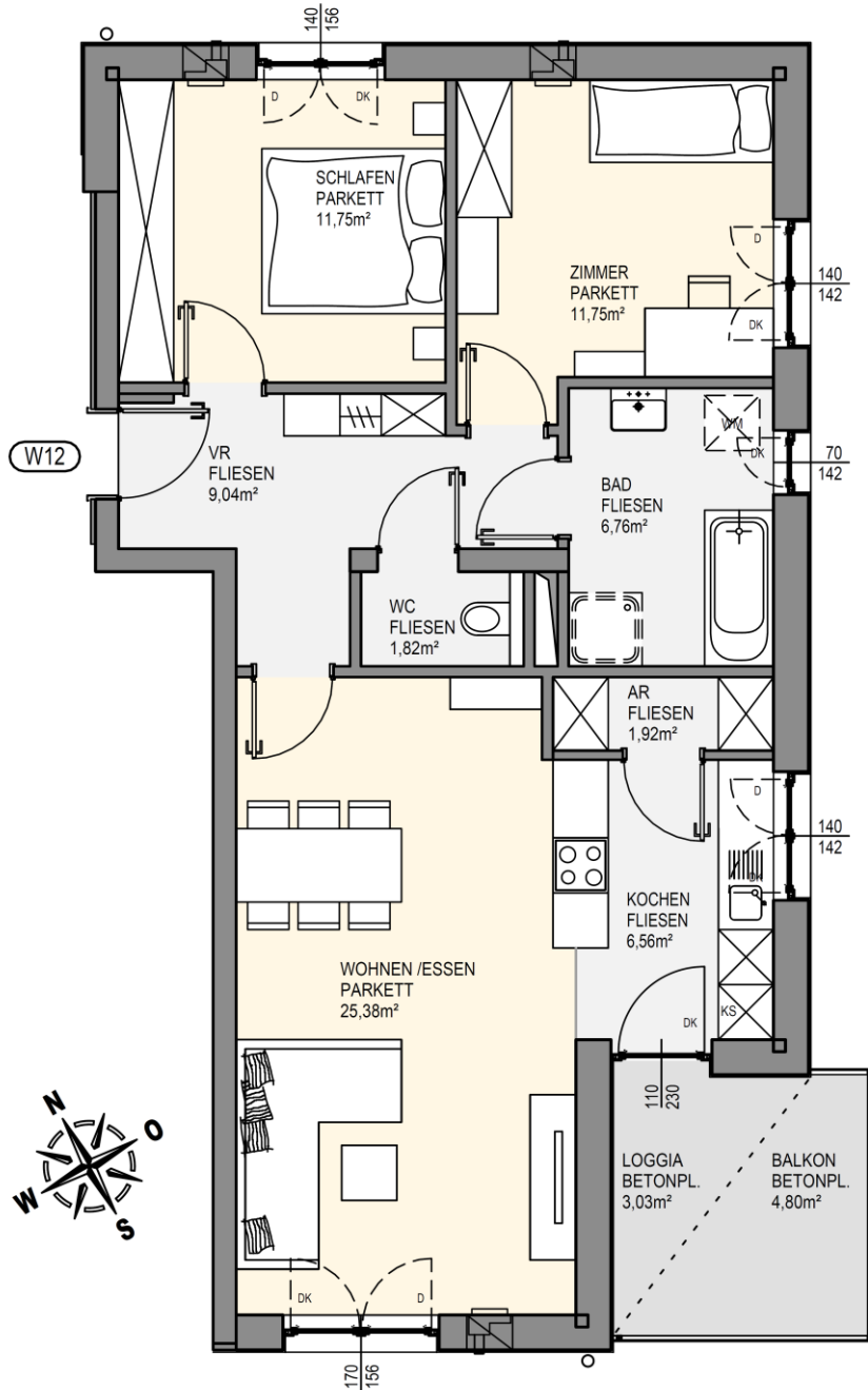
Übersichtsplan
