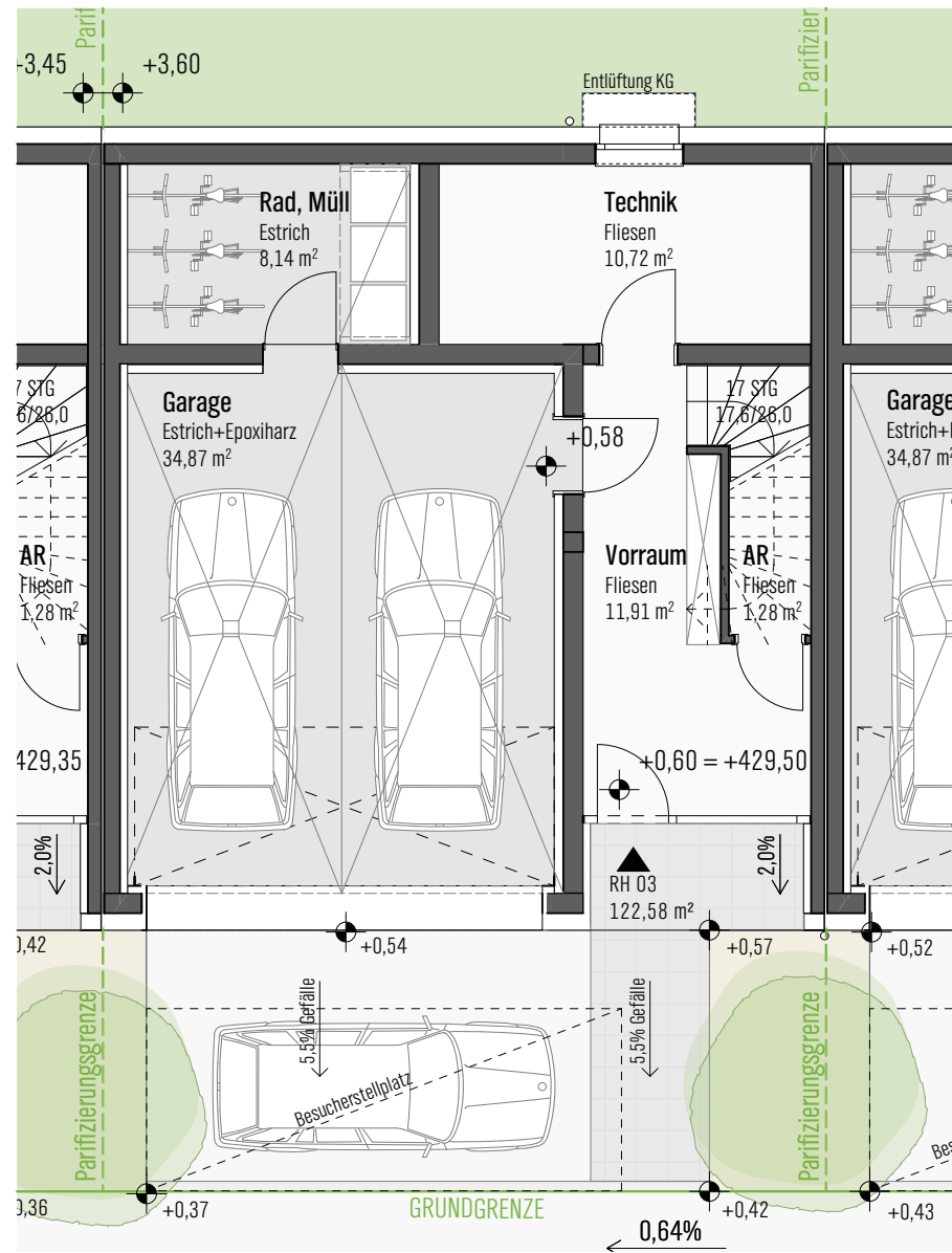
KG M 1:100
