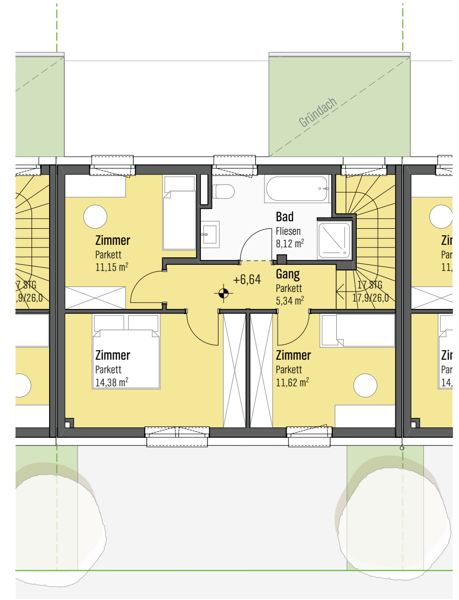
1.OG 1:100
