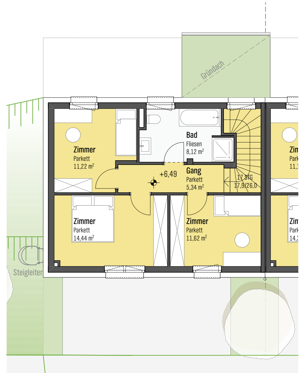
1.OG 1:100
