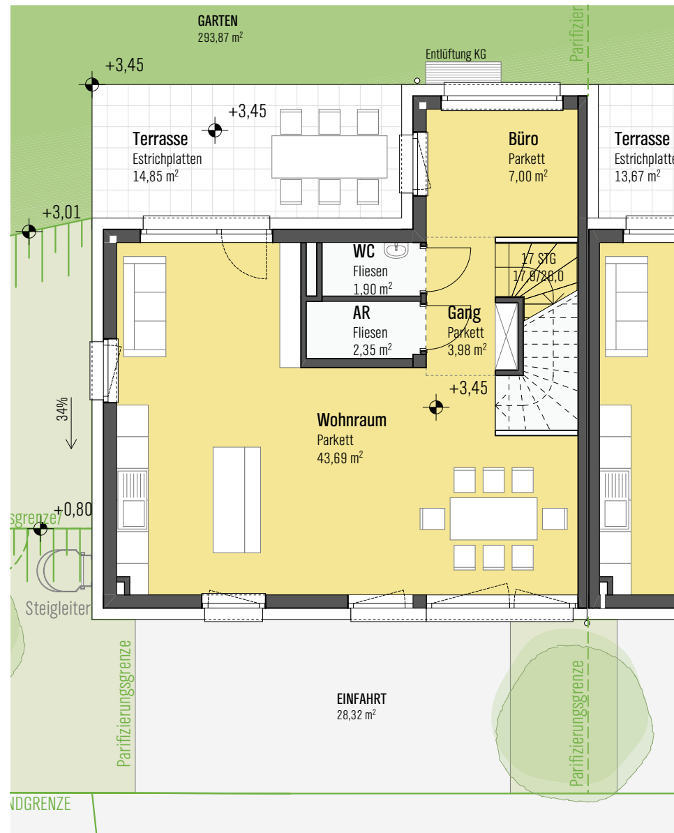
EG M 1:100
