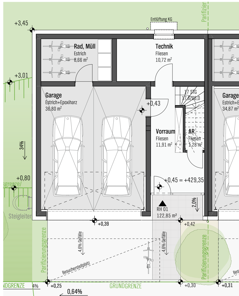
KG M 1:100
