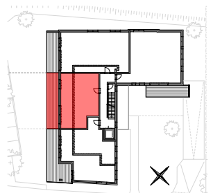
Lageplan 2.OG
