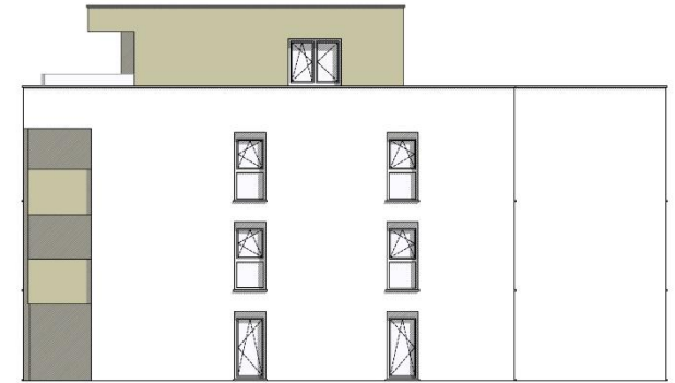
Ansicht OST
