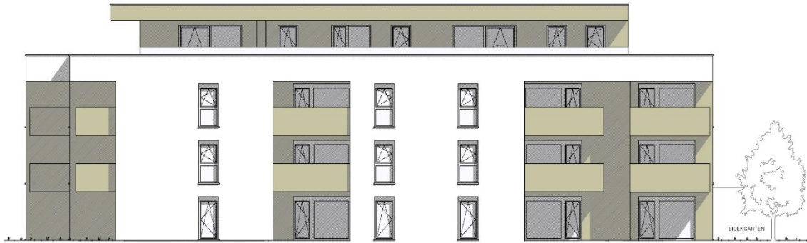
Ansicht SÜD
