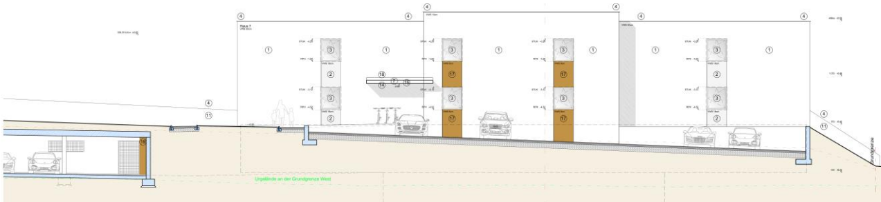
Ostansicht
