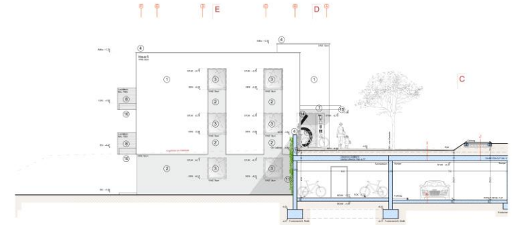
Südansicht
