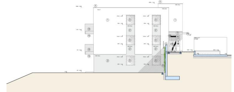
Südansicht
