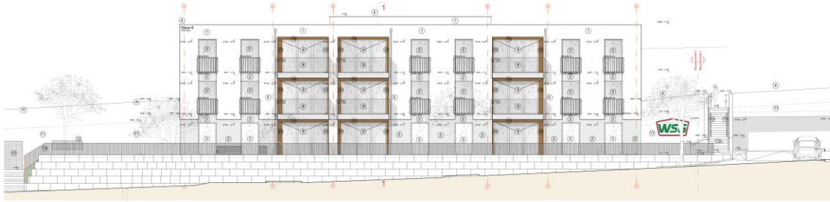
Westansicht
