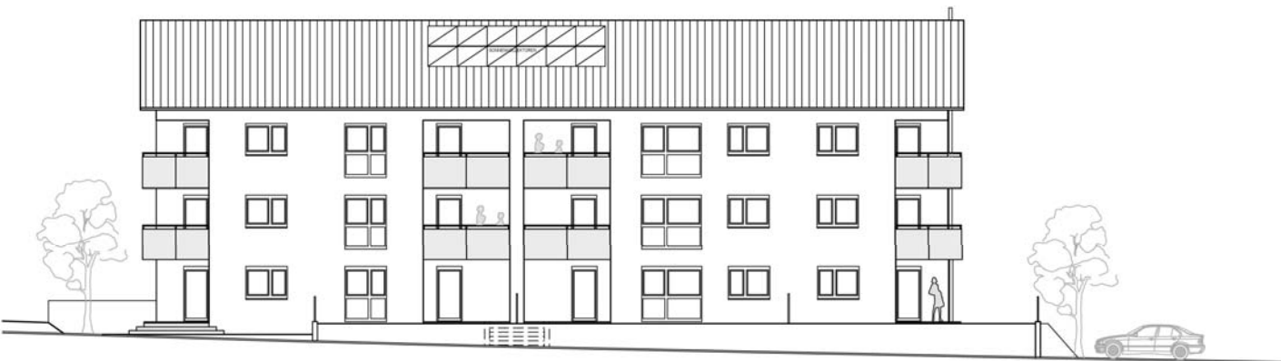
Südansicht
